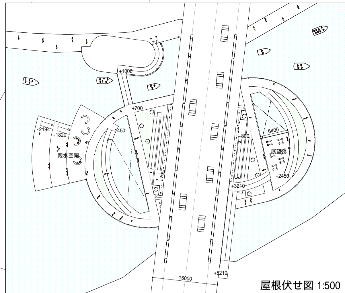
屋根伏せ図 1:500
