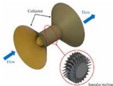
図1 衝動タービンと集流装置を組み合わせた潮流発電装置
