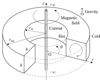
図 1 解析モデル
