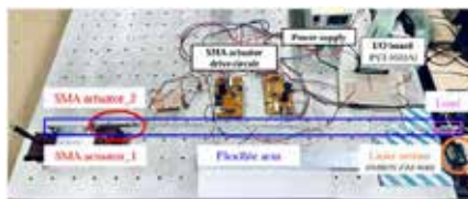
図 2. 形状記憶合金アクチュエータを用いた柔軟ビームの振動制御例(3-4)
