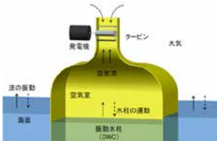
図 3 振動水柱型波力発電プラント
