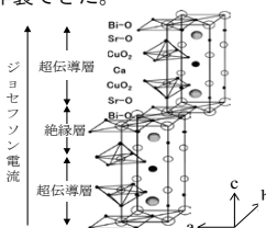
図 1 Bi 系高温超伝導体の結晶構造
