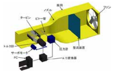
図 4 風洞試験装置概略図
