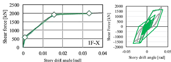
図Ⅰ 解析モデル設定・解析結果の検証
