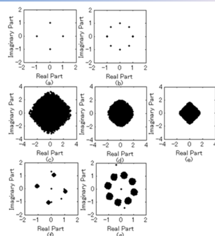
(a), (b) : 入力信号 (4-PSK と 8-PSK) (c), (d), (e) : 観測信号 (チャネル出力) (f), (g) : 復元信号 図1 無線通信への応用 (2入力3出力の場合)
