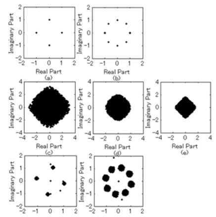
(a), (b) : 入力信号 (4-PSK と 8-PSK) (c), (d), (e) : 観測信号 (チャネル出力) (f), (g) : 復元信号 図1 無線通信への応用 (2入力3出力の場合)
