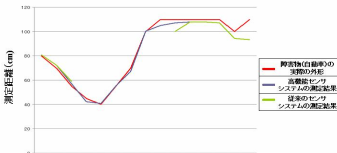
図1 自動車ソナーとしての測定性能
