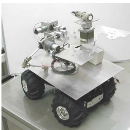
写真1 水平維持機構を搭載した移動ロボット
