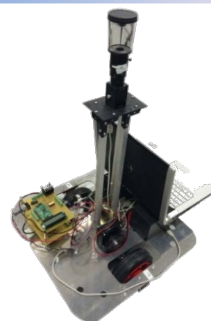
写真2 全方位カメラを搭載した移動ロボット
