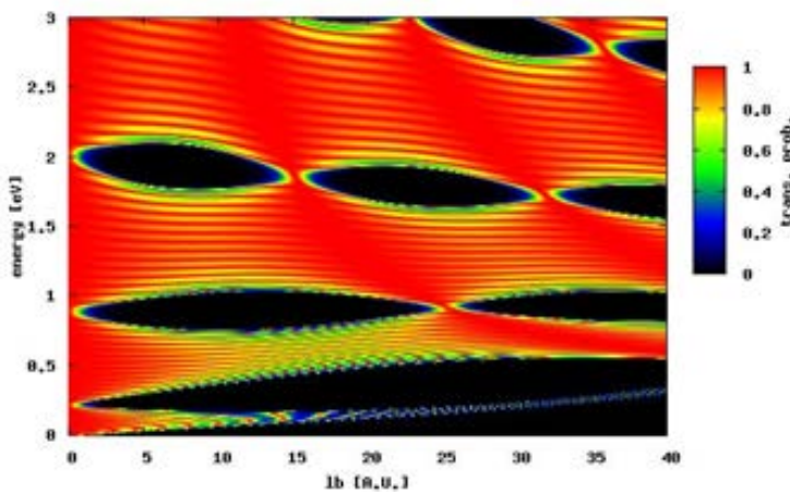
図1 半導体超格子のバンド構造例
