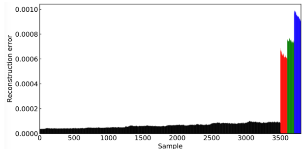
図 1 AE センシングとオートエンコーダにより異常度を算出した結果 (黒: 正常データ, 赤: 異常(1), 緑: 異常(2), 青: 異常(3))
