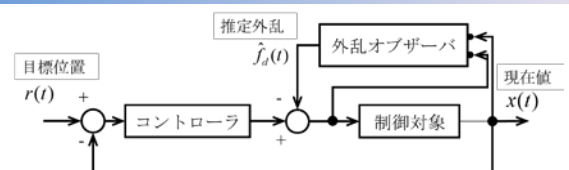
状態推定器を併用したサーボ制御
