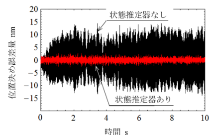
位置決め精度の実験結果
