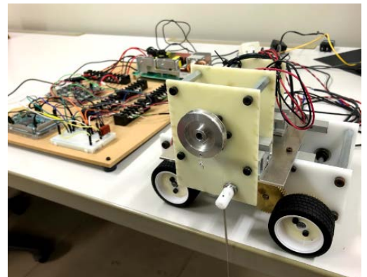
図 台車クレーン実験装置
