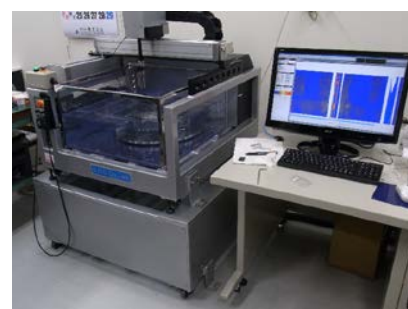
超音波探傷映像化装置 SDS-WIN4400R
