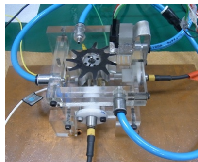
軸受内径 3mm 直交 2 軸油膜厚さ測定 実験装置写真
