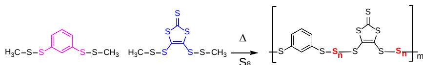
無溶媒合成反応による正極活物質の合成
