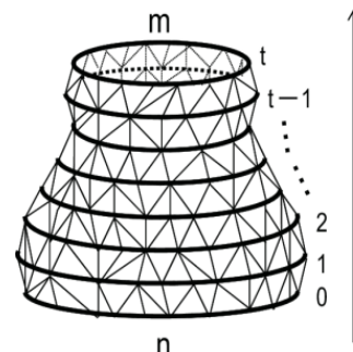
図1: 離散化された時空内での弦の伝播
