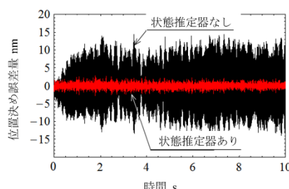
位置決め精度の実験結果
