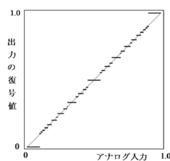
図4 入出力特性
