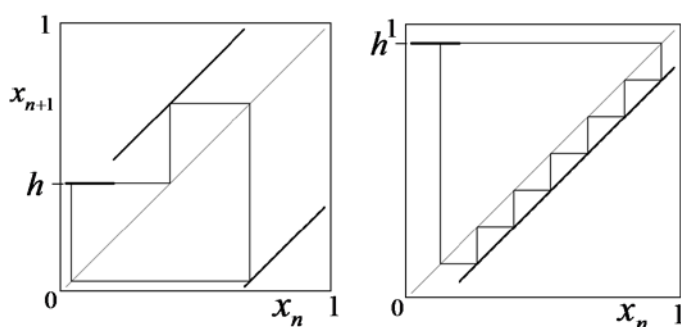
図3 1次元差分方程式と超安定周期軌道
